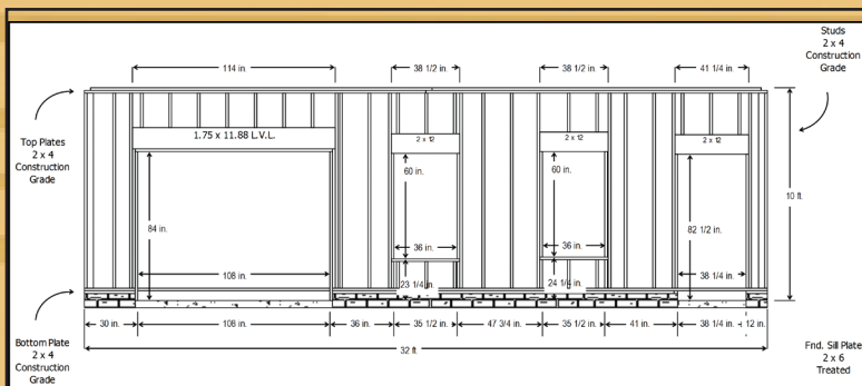
STUD FRAMING LAYOUTS
